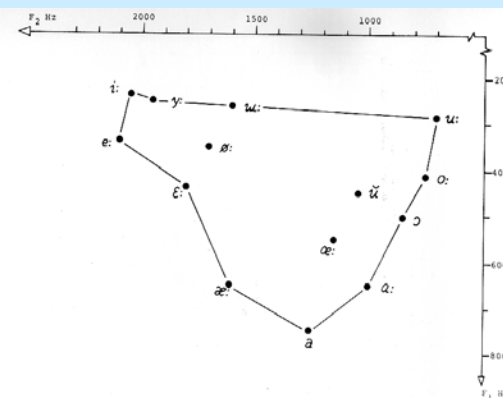
Figur 5. Akustiskt vokaldiagram med svenska vokaler. Formantvärden från Fant.
